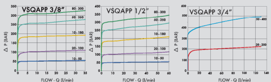
PRESSIONE/PORTATA PRESSURE/FLOW
